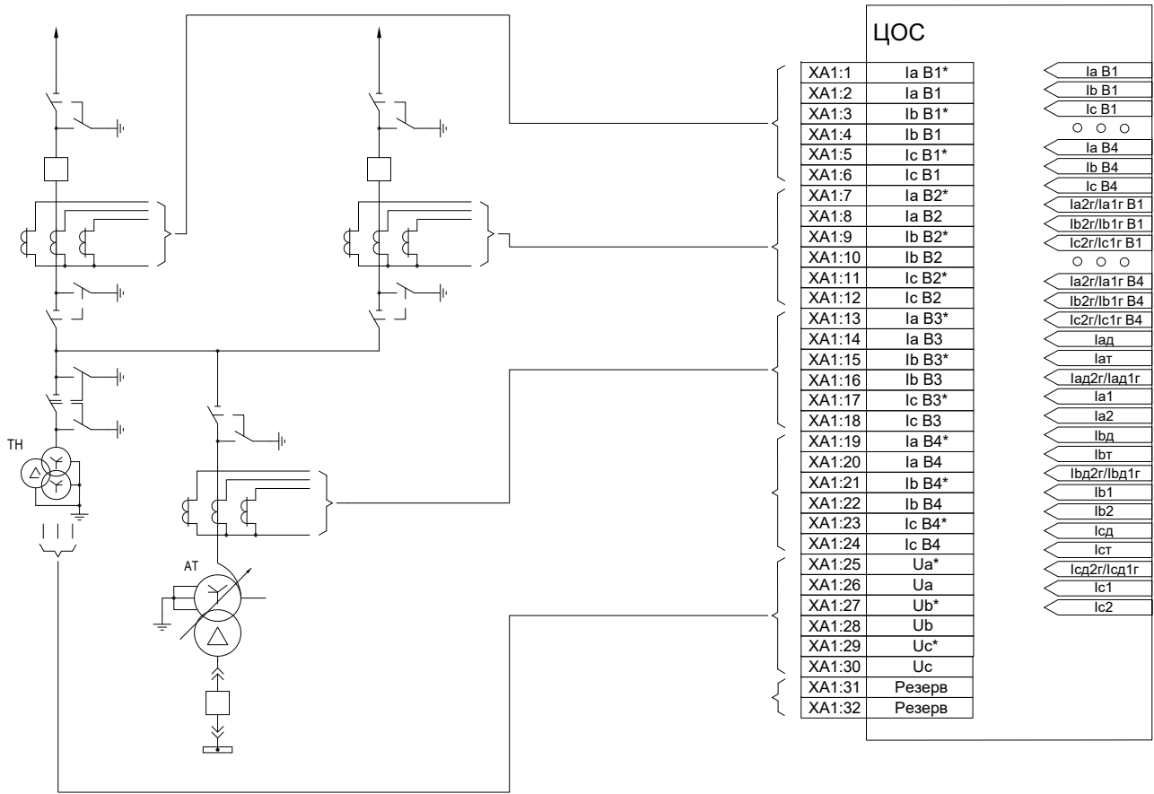
Рисунок Б.1 – Вариант подключения аналоговых цепей ТТ и ТН к устройству
